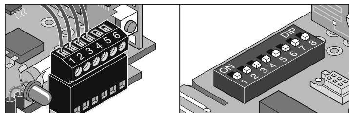
Klemme 1 + 2 Anschluss für Taster 2, nur wenn DIP-Schalter 2 ON
