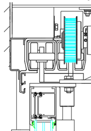
Laufschiene
