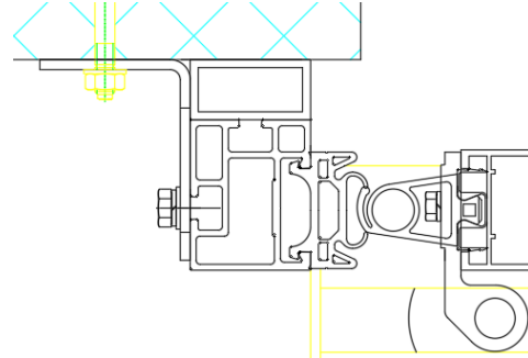
Befestigung am Mauerwerk und Torstockdichtung
