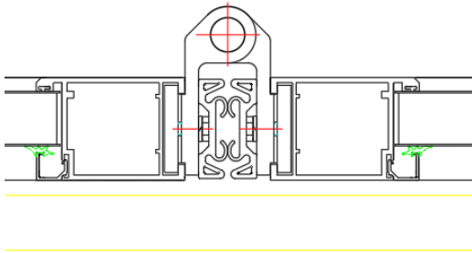
Flügeldichtung
