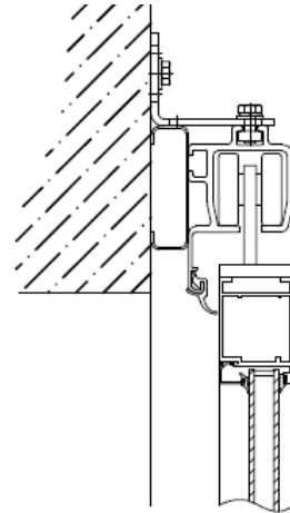
Laufschiene
