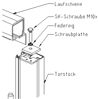
Laufschienenverschraubung
